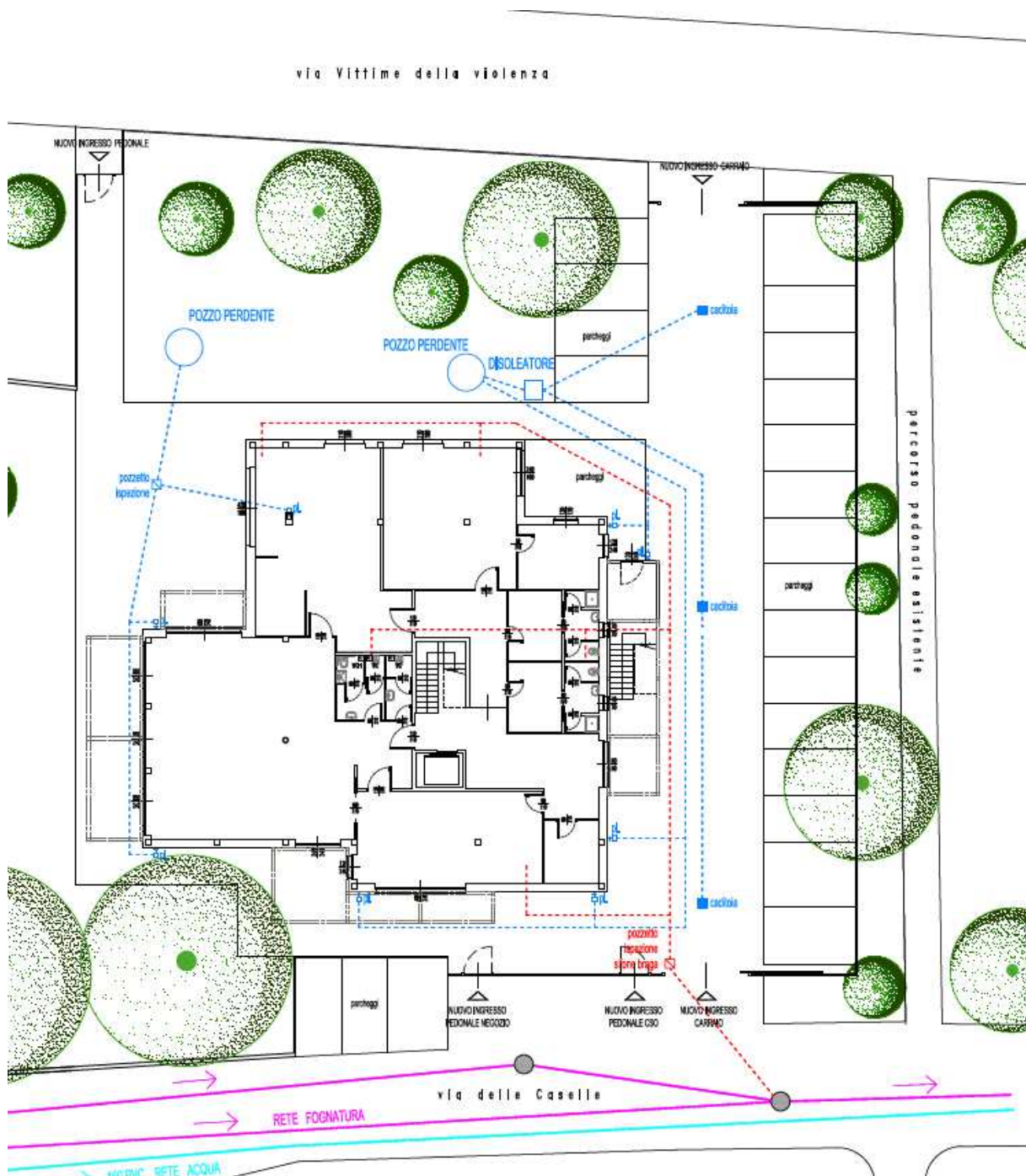
Figura 8 – Estratto dalla tavola di PA tav 9.1_schema reti esterne
