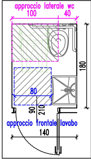
BAGNO DISABILI P.NO 1°/2°
