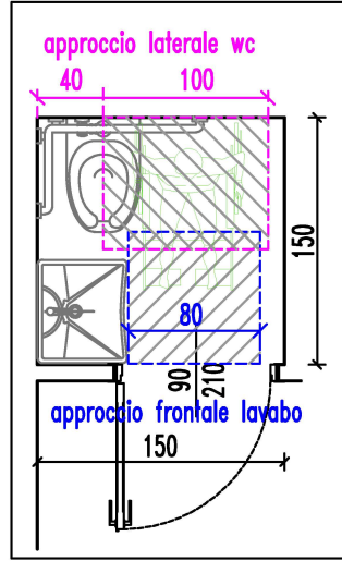
BAGNO DISABILI P.NO TERRA
