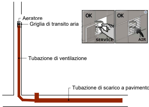
PARTICOLARE VENTILAZIONE TUBAZIONE DI SCARICO
