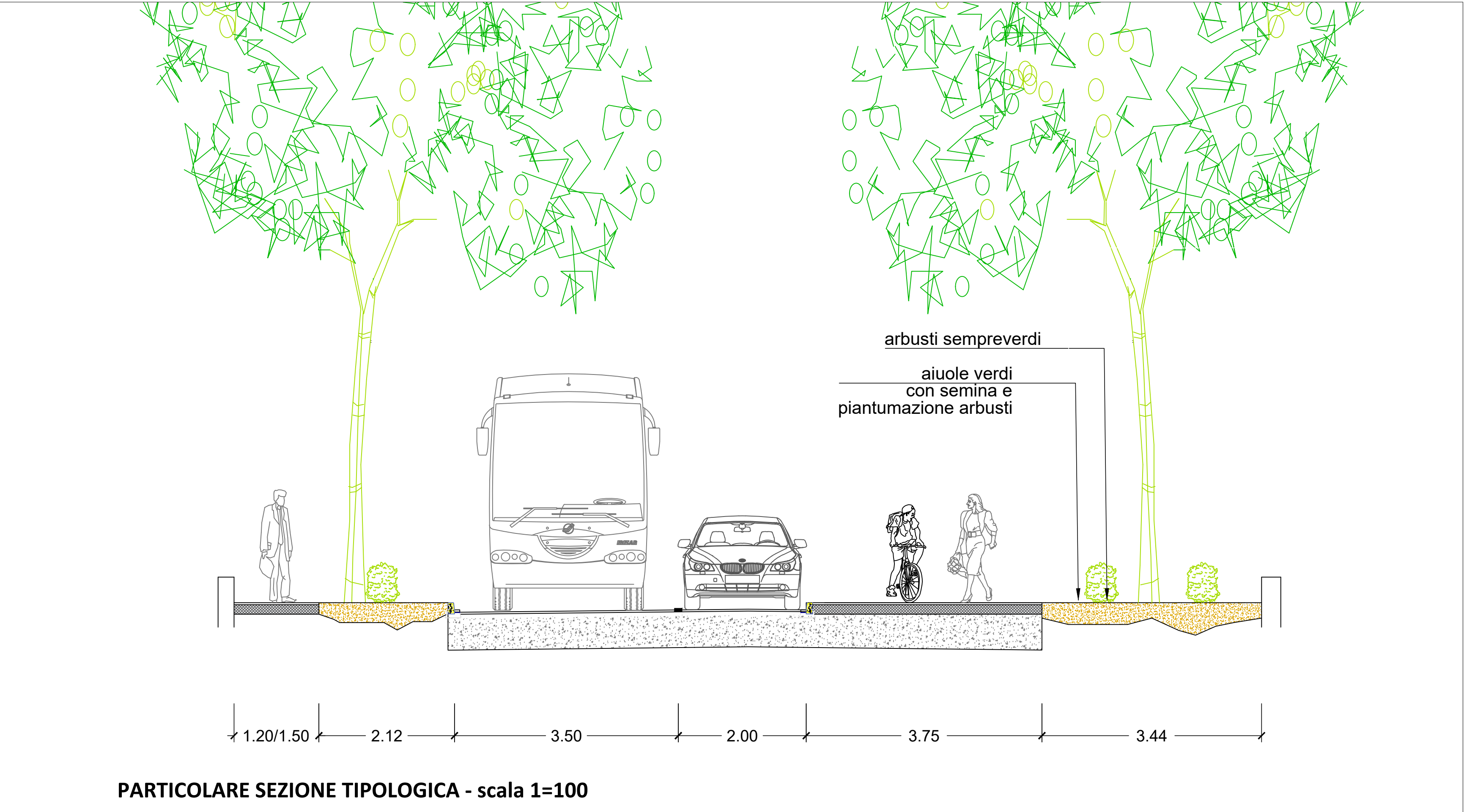
PARTICOLARE SEZIONE TIPOLOGICA - scala 1=100
