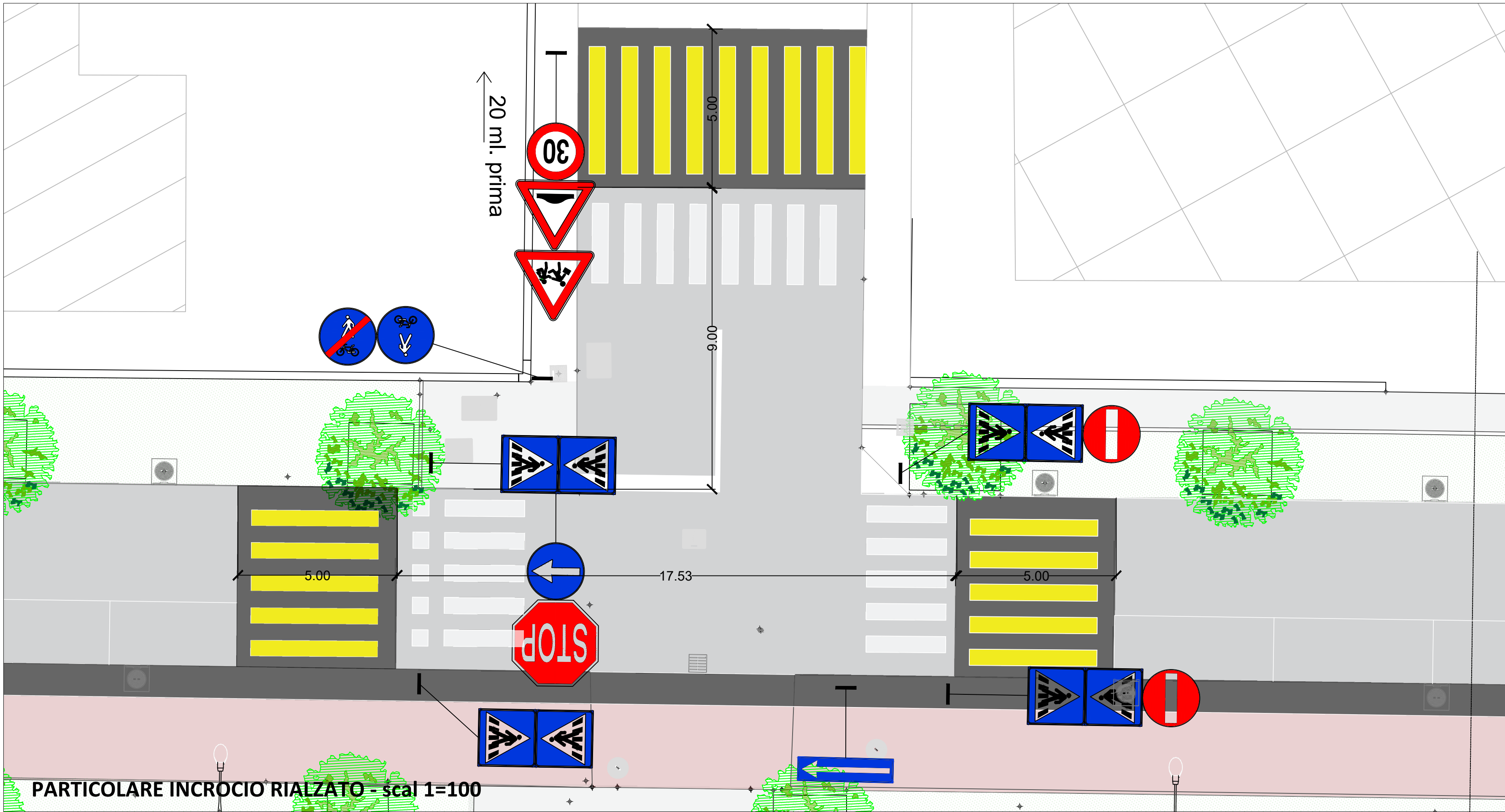
PARTICOLARE INCROCIO RIALZATO - scala 1=100
