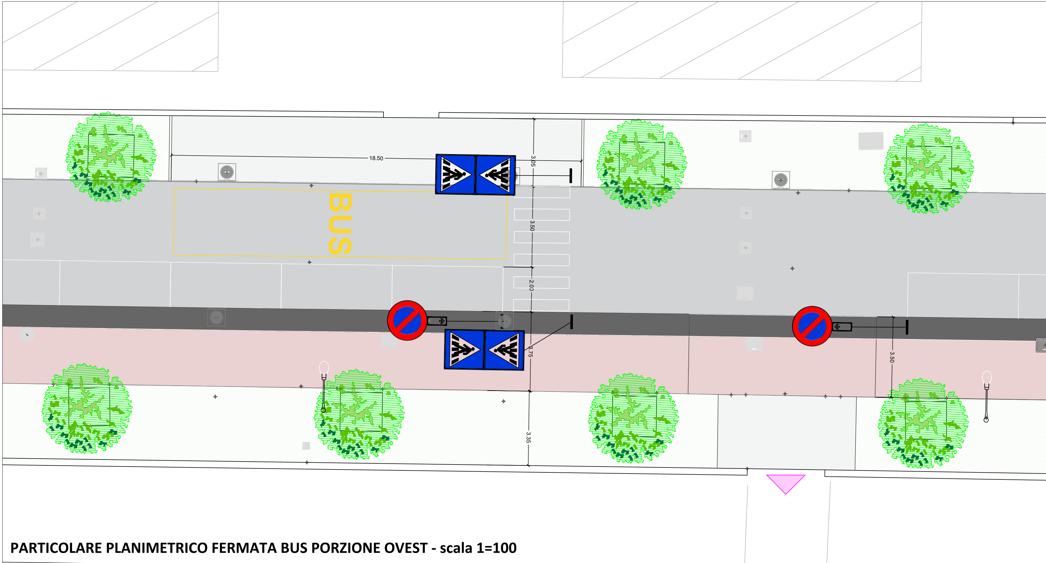
PARTICOLARE PLANIMETRICO FERMATA BUS PORZIONE OVEST - scala 1=100
