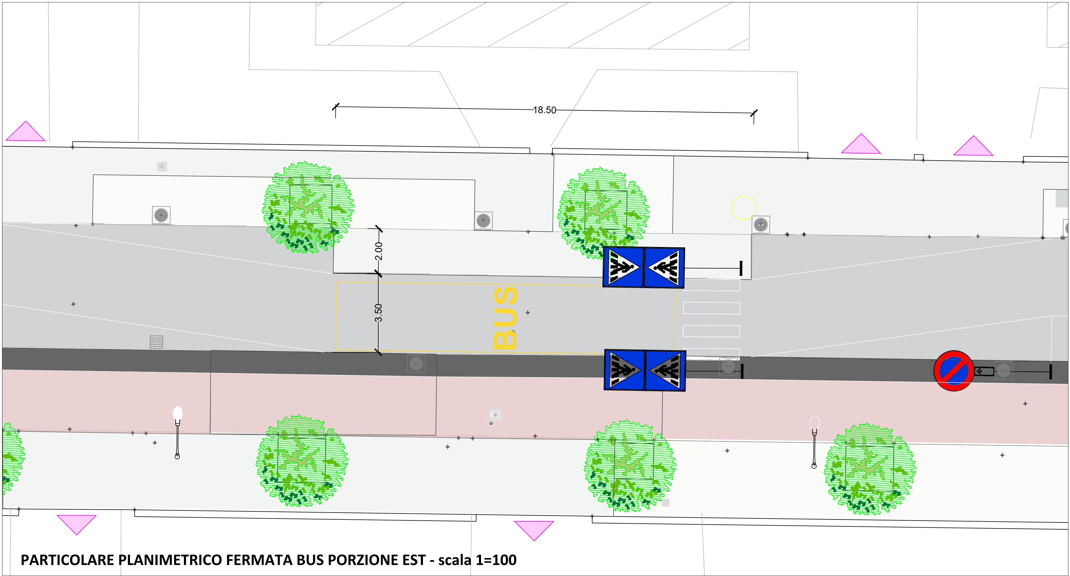
PARTICOLARE PLANIMETRICO FERMATA BUS PORZIONE EST - scala 1=100
