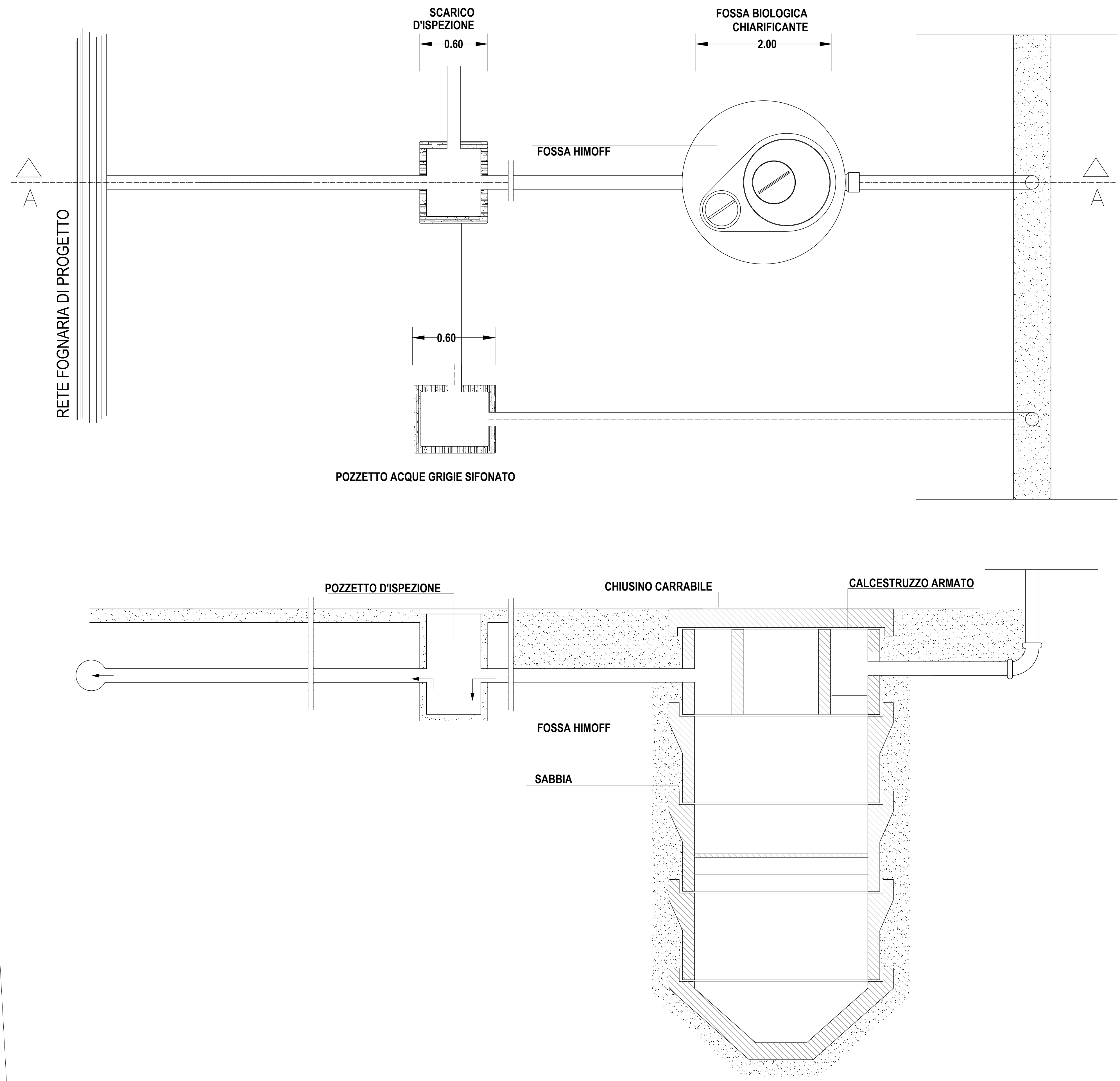
SCHEMA IMPIANTO FOGNARIO SCARICHI DOMESTICI
