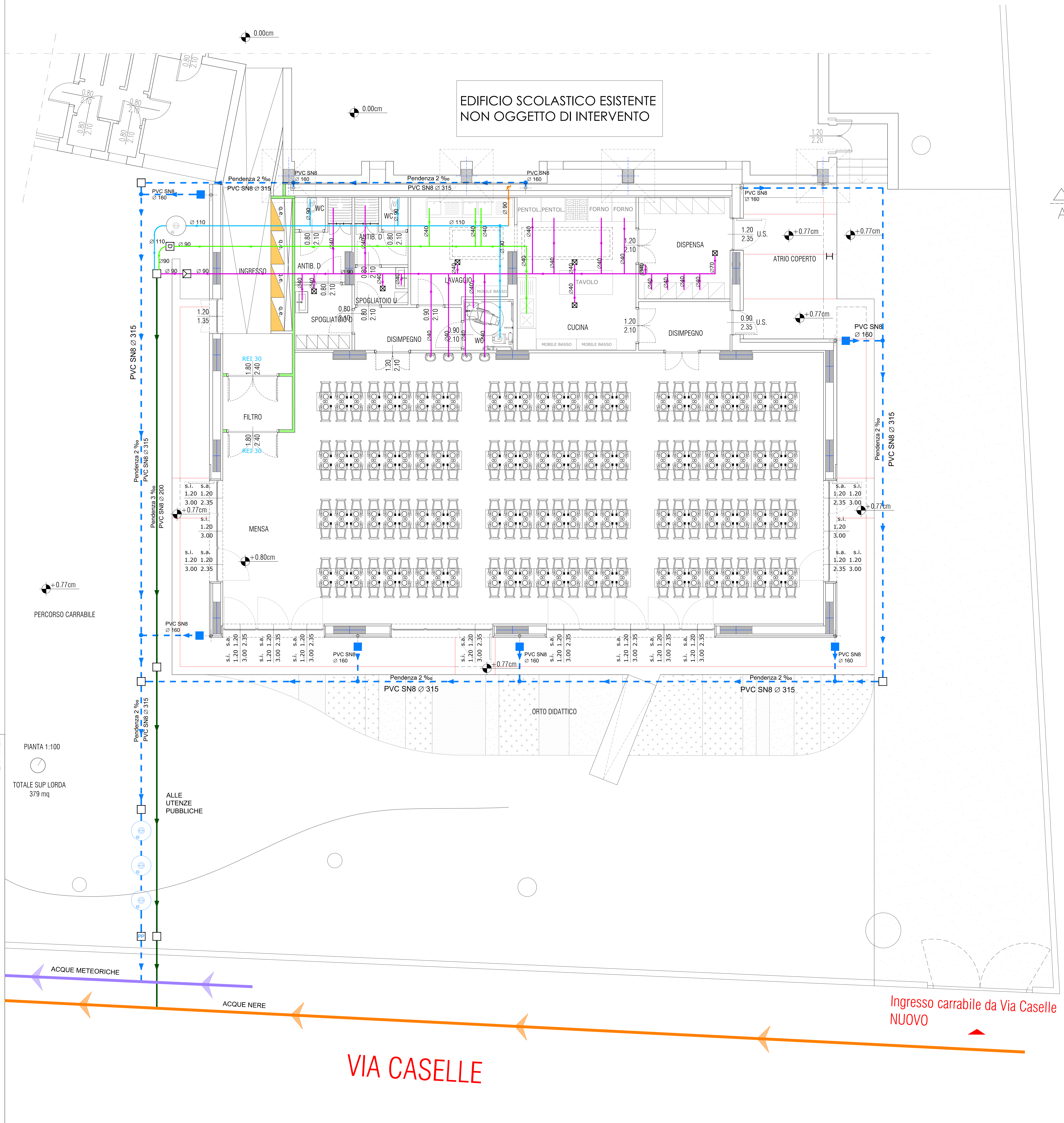
SCHEMA IMPIANTO FOGNARIO SCARICHI DOMESTICI
