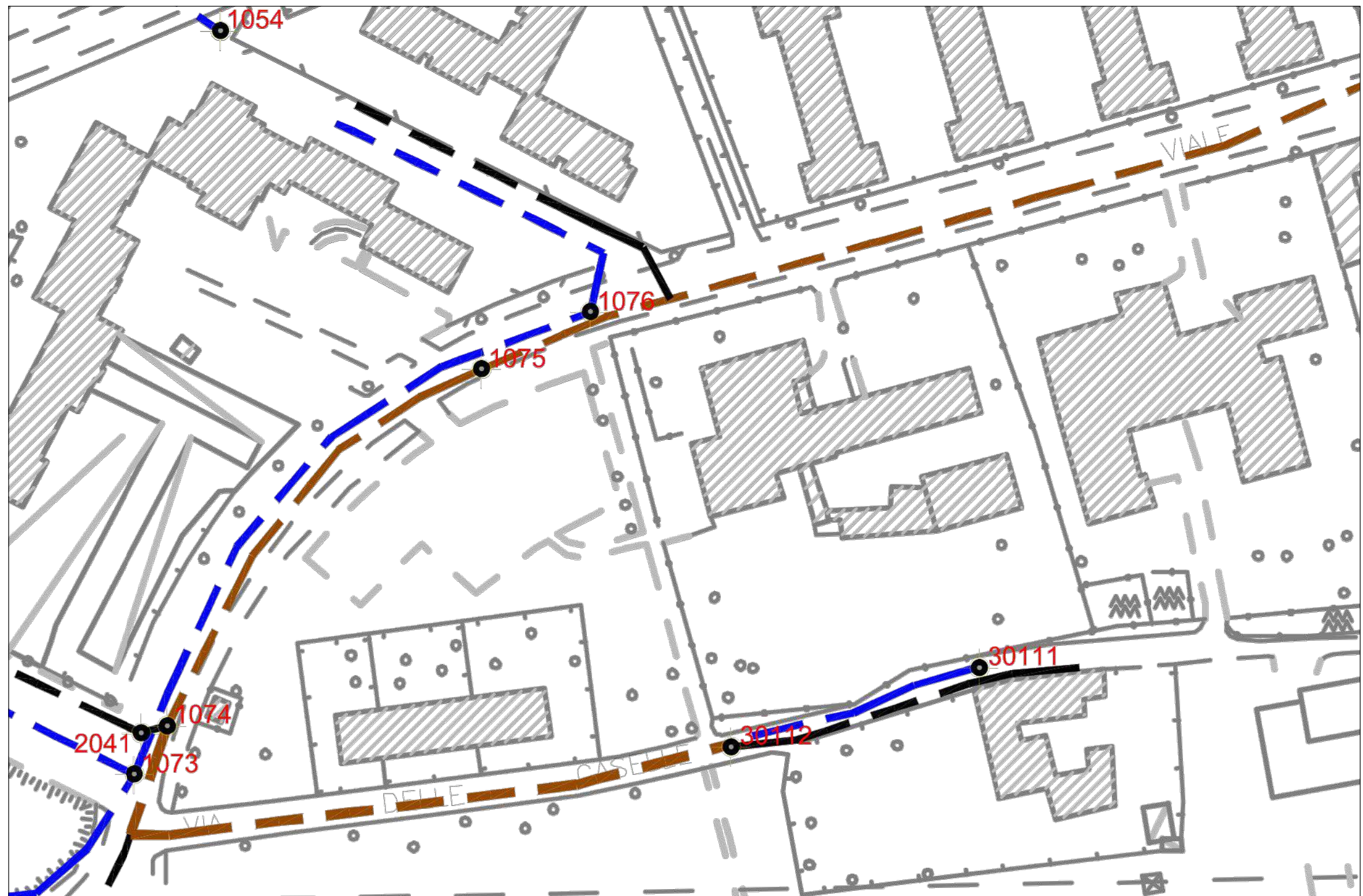
PLANIMETRIA RETE FOGNARIA COMUNALE - SCALA 1:1000
