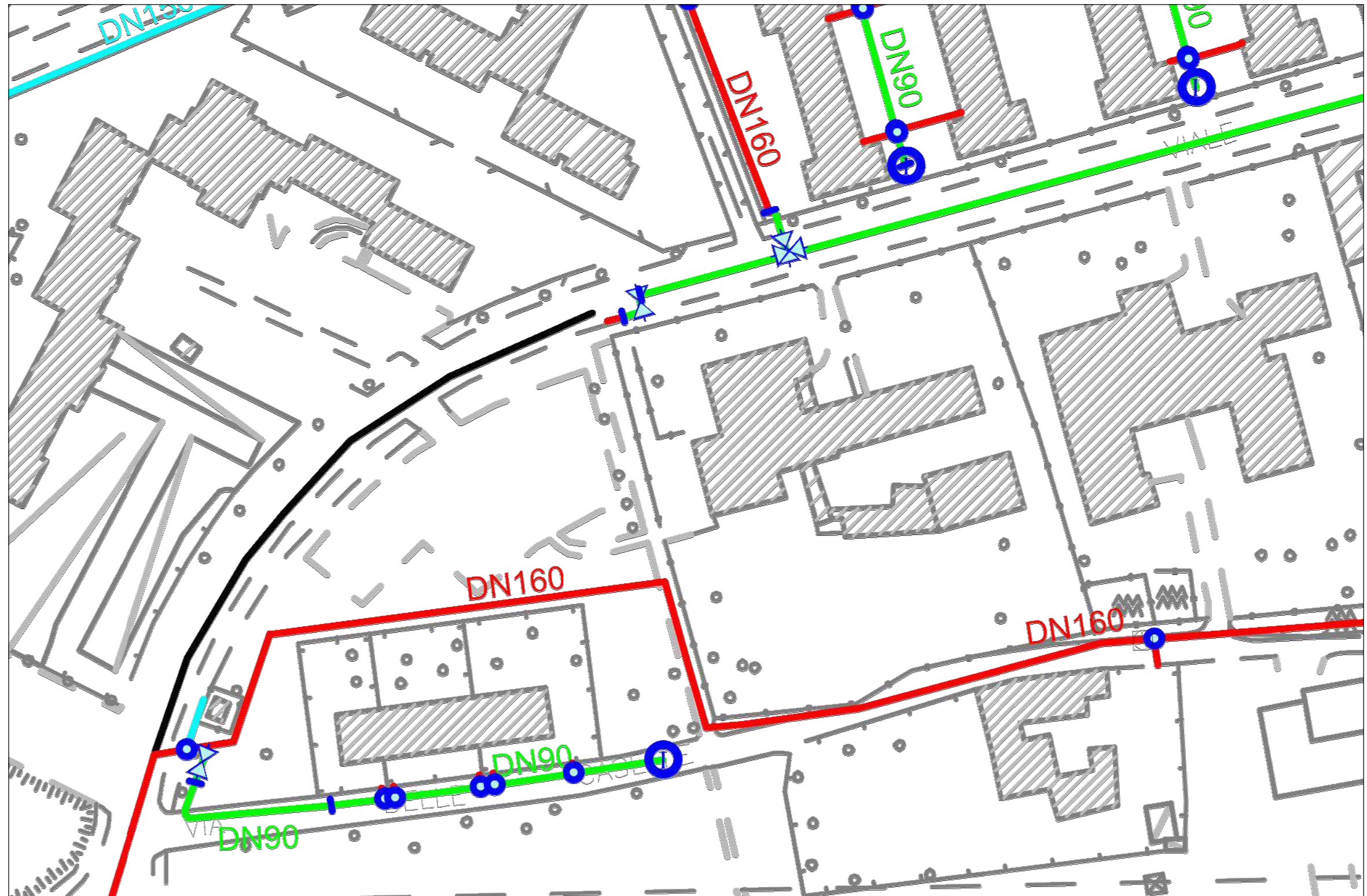
PLANIMETRIA RETE ACQUEDOTTO COMUNALE - SCALA 1:1000
