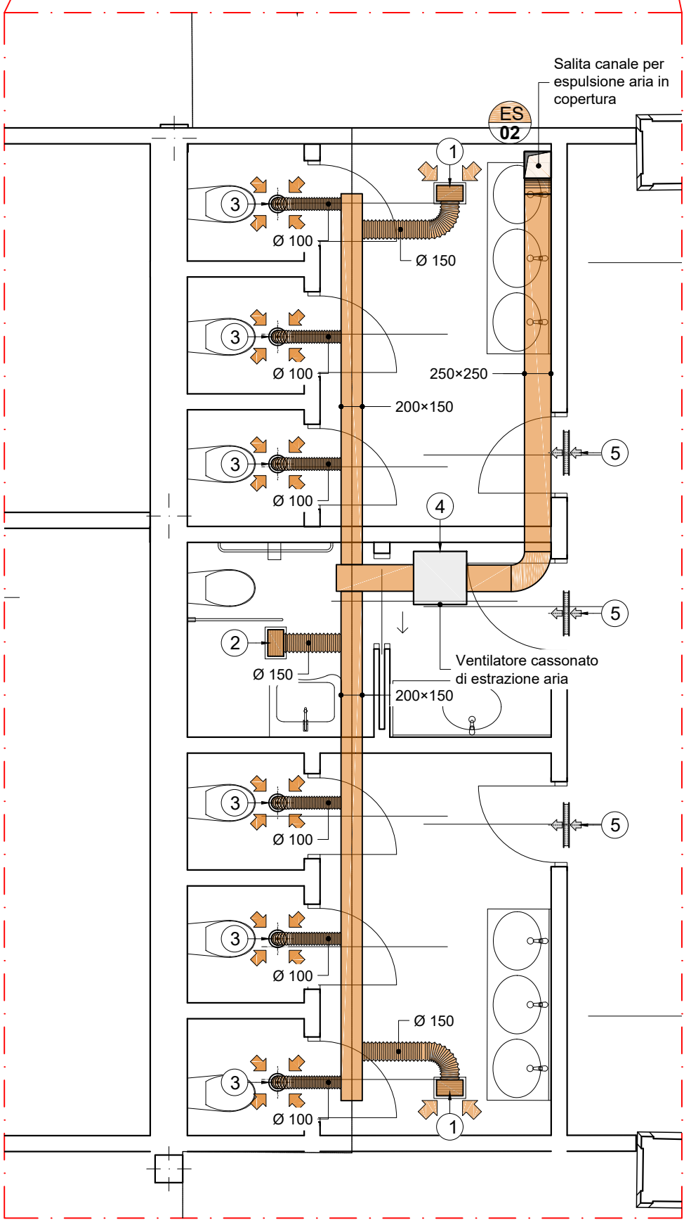
BLOCCO SERVIZI 2 scala 1:50
