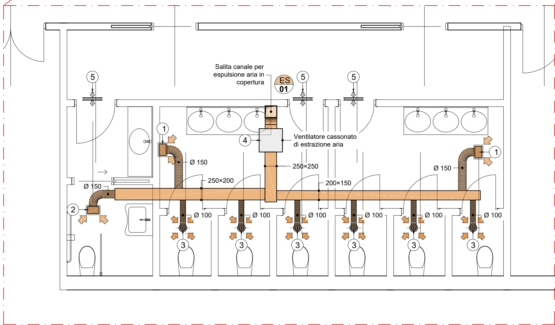
BLOCCO SERVIZI 1 scala 1:50
