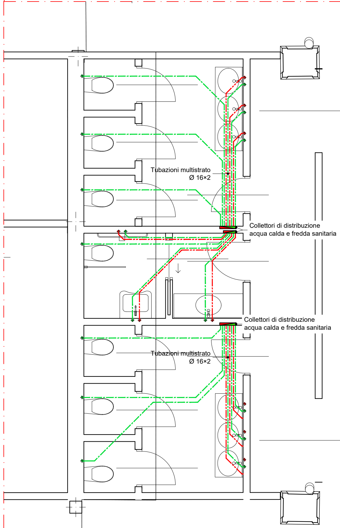
BLOCCO SERVIZI 2 scala 1:50
