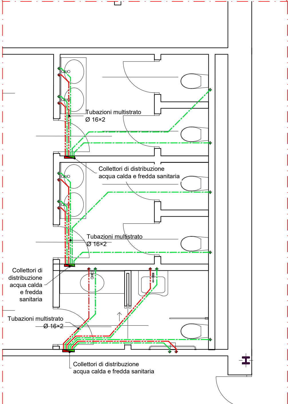
BLOCCO SERVIZI 3 scala 1:50
