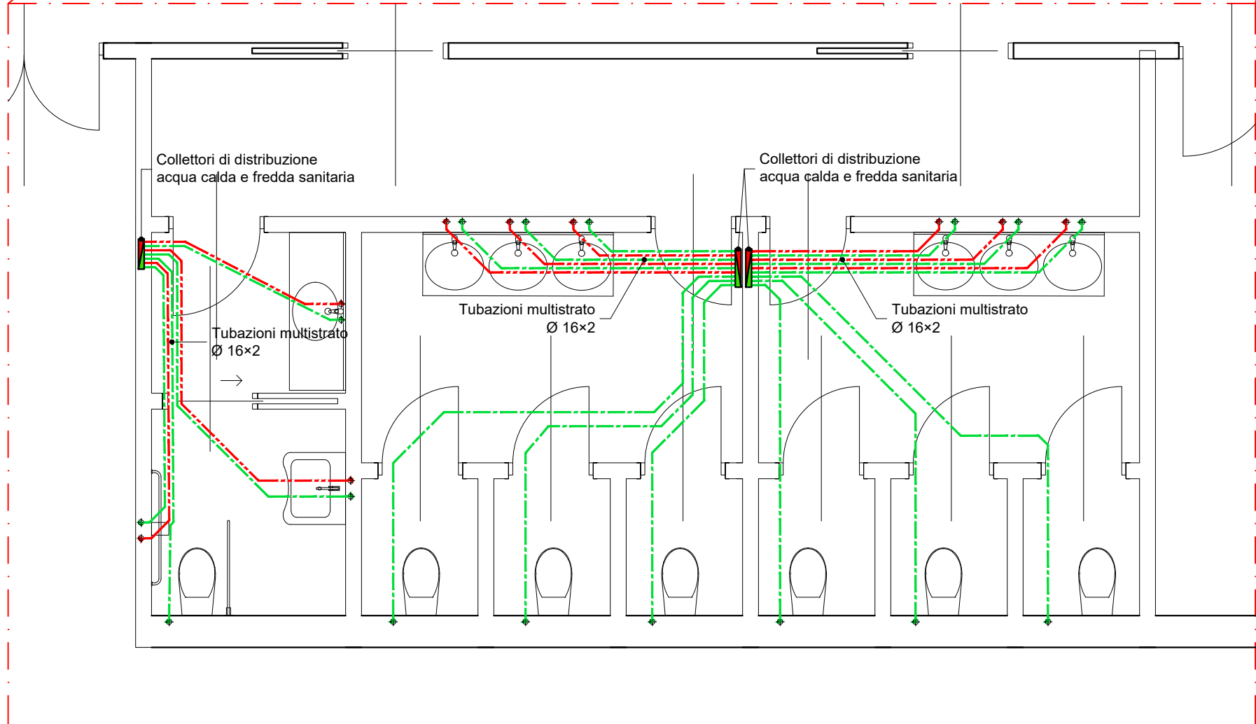
BLOCCO SERVIZI 1 scala 1:50
