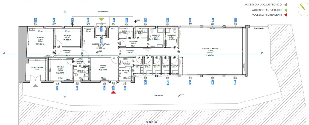
Pianta Piano Terra Stato di Fatto
