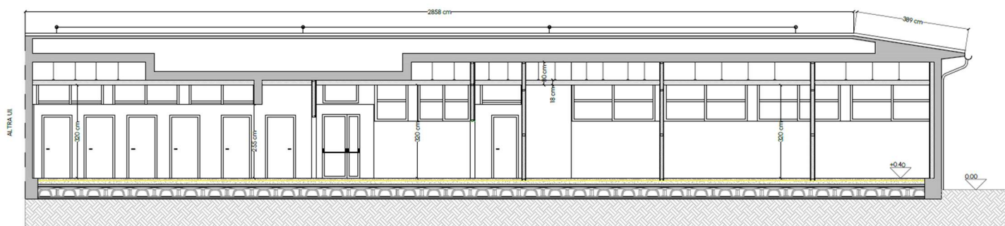
Sezione longitudinale Stato di Progetto
