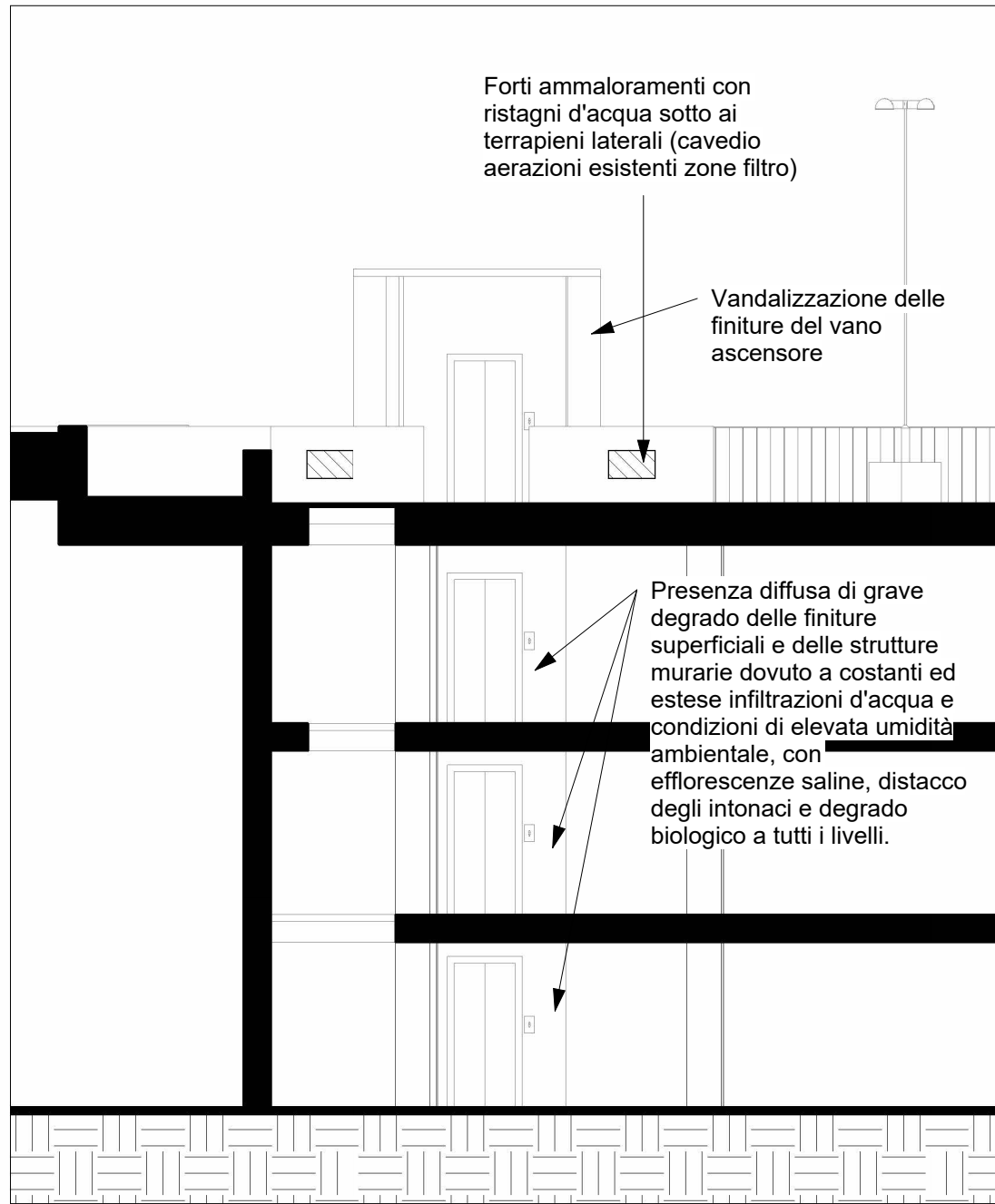
SEZIONE TIPOLOGICA - AMMALORAMENTI
