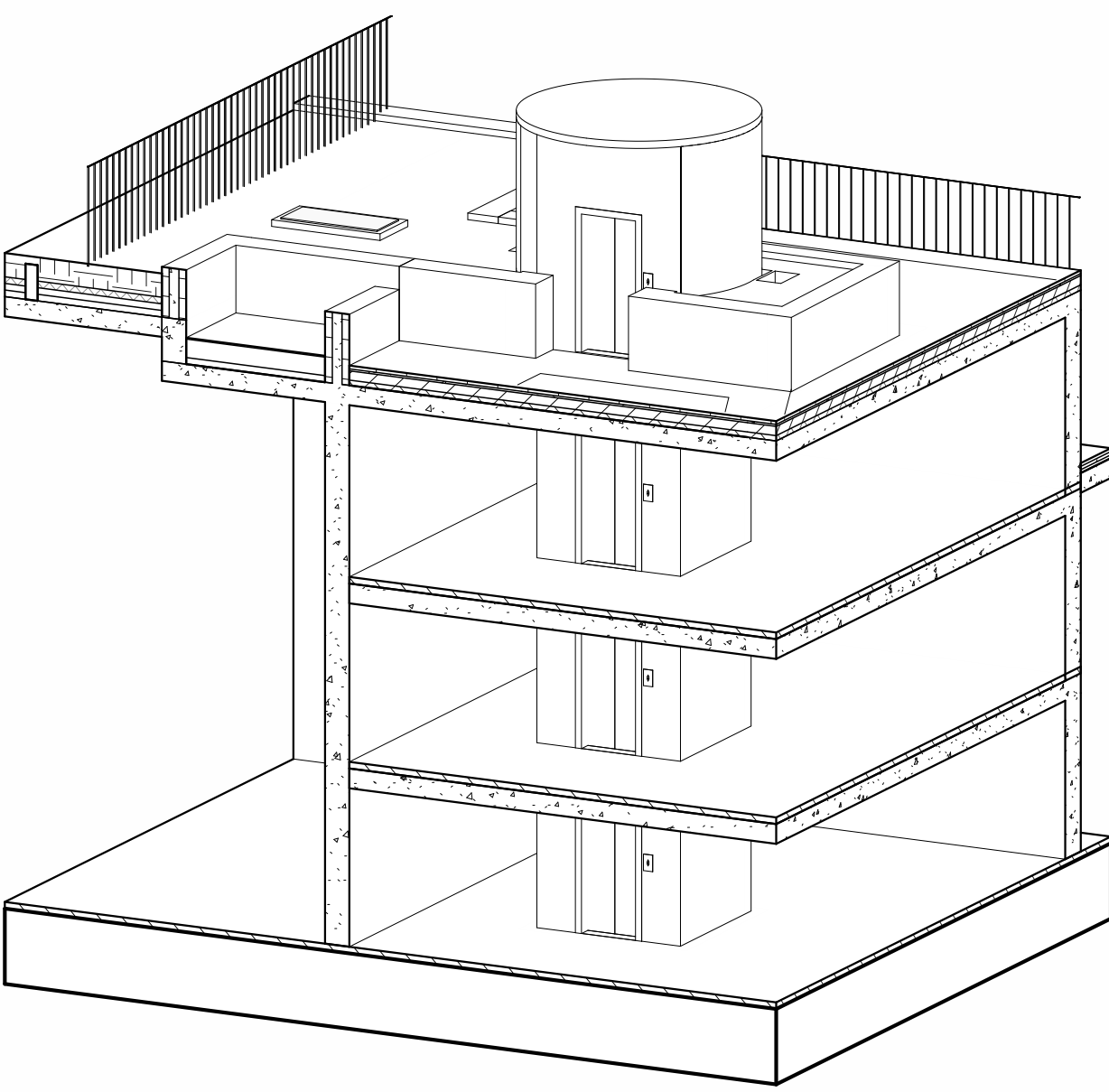
SPACCATO 3D - STATO DI FATTO
