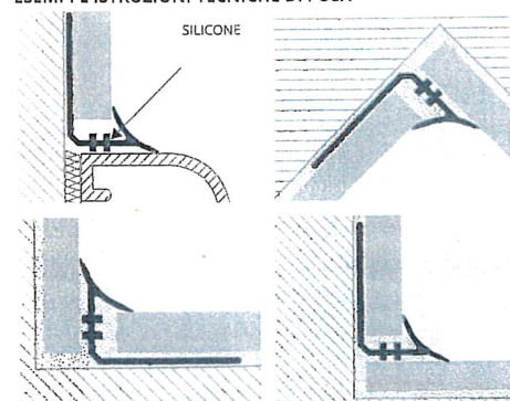
RACCORDI ANGOLI INTERNI, ESTERNI e TRE VIE PROINTER ALLUMINIO ANODIZZATO ARGENTO (AA) e ORO (AO) - conf. 2 PZ
