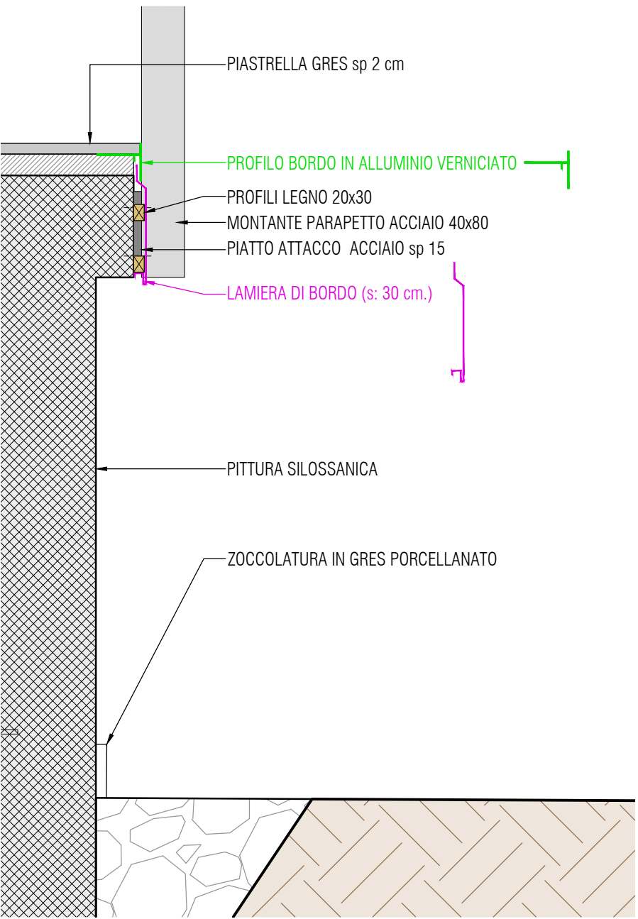
SEZIONE TIPO BORDO TERRAZZO PISCINA SCALA 1:10
