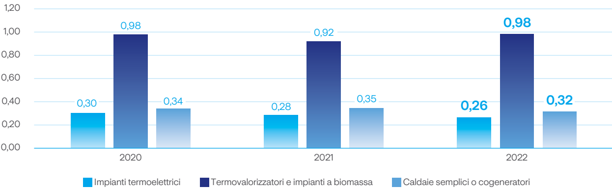
Figura 44 Acqua utilizzata per unità di energia prodotta (m³/MWh)
